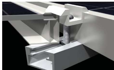
Exemple B: aile de serrage
