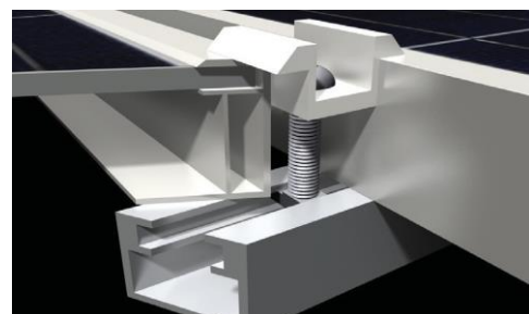
Beispiel B: Klemmflügel
