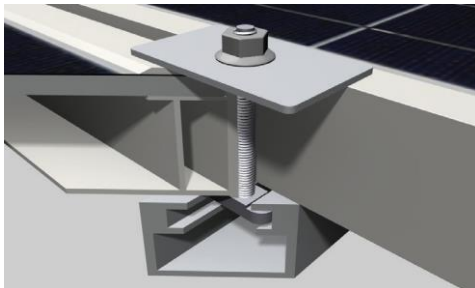
Voorbeeld A: klemplaat
