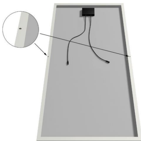
La borne de terre doit être fixée sur l'un des trous de mise à la terre prévus et repérés au dos du cadre des modules.
